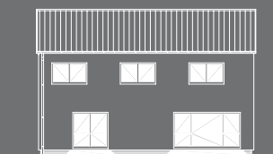
POHLED ZADNÍ
